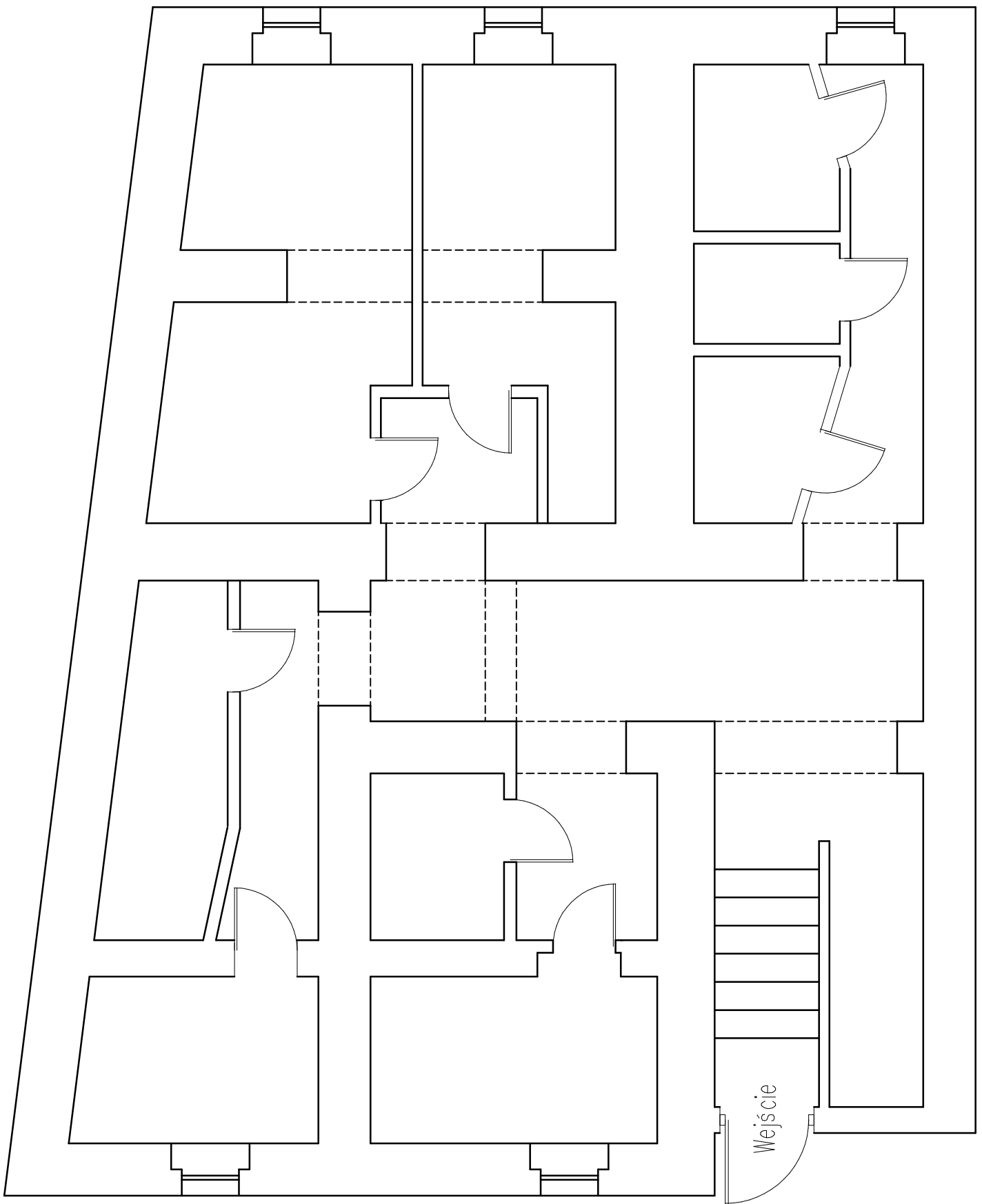
INWENTARYZACJA – RZUT PIWNIC BUDYNEK UL. CHROBREGO 16 SKALA: 1–50 Papier Format A4 OPRACOWAŁ: JÓZEF BIENIARZ
