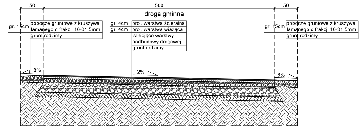
PRZEKRÓJ POPRZECZNY ODNOGI (OD KM 0+000 DO KM 0+061) ODCINKA GŁÓWNEGO DROGI W KM 101,5
