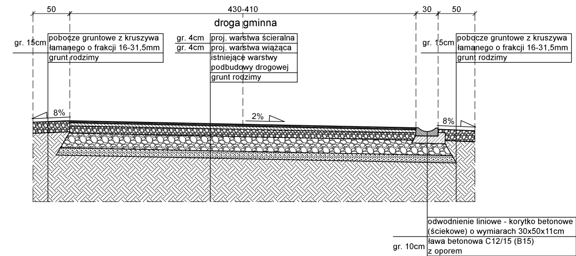
PRZEKRÓJ POPRZECZNY ODNOGI (OD KM 0+000 DO KM 0+062) ODCINKA GŁÓWNEGO DROGI W KM 308,5
