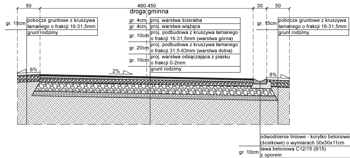
PRZEKRÓJ POPRZECZNY ODCINKA GŁÓWNEGO DROGI OD KM 0+308,5 DO KM 0+453
