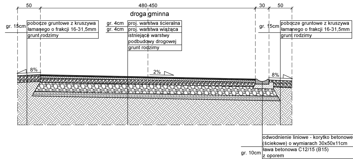
PRZEKRÓJ POPRZECZNY ODCINKA GŁÓWNEGO DROGI OD KM 0+000 DO KM 0+308,5
