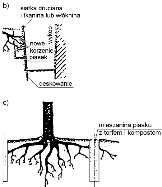
a) przekrój ogólny, b) szczegół wykopu, c) wstępna faza zabezpieczenia, wykonywana najlepiej przed właściwym wykopem
