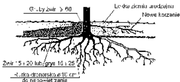
Rys. 4. Pień drzewa obsypany na wysokość 0,2 ÷ 0,5 m ze specjalnymi napowietrzającymi warstwami zwirowymi (wg [10])
