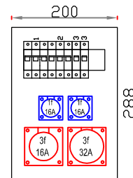
Elewacja rozd. stacjonarnej - PCE IP44
