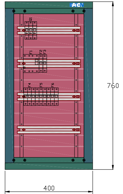
Elewacja rozd. natynkowej R2 IP30
