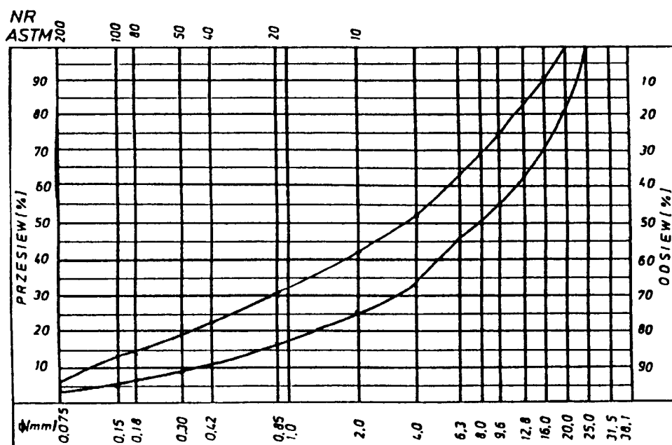
Rys. 11. Krzywe graniczne uziarnienia mieszanki mineralnej 0+25 mm do warstwy wiążącej, wyrównawczej i wzmacniającej z betonu asfaltowego dla KP 2-6
