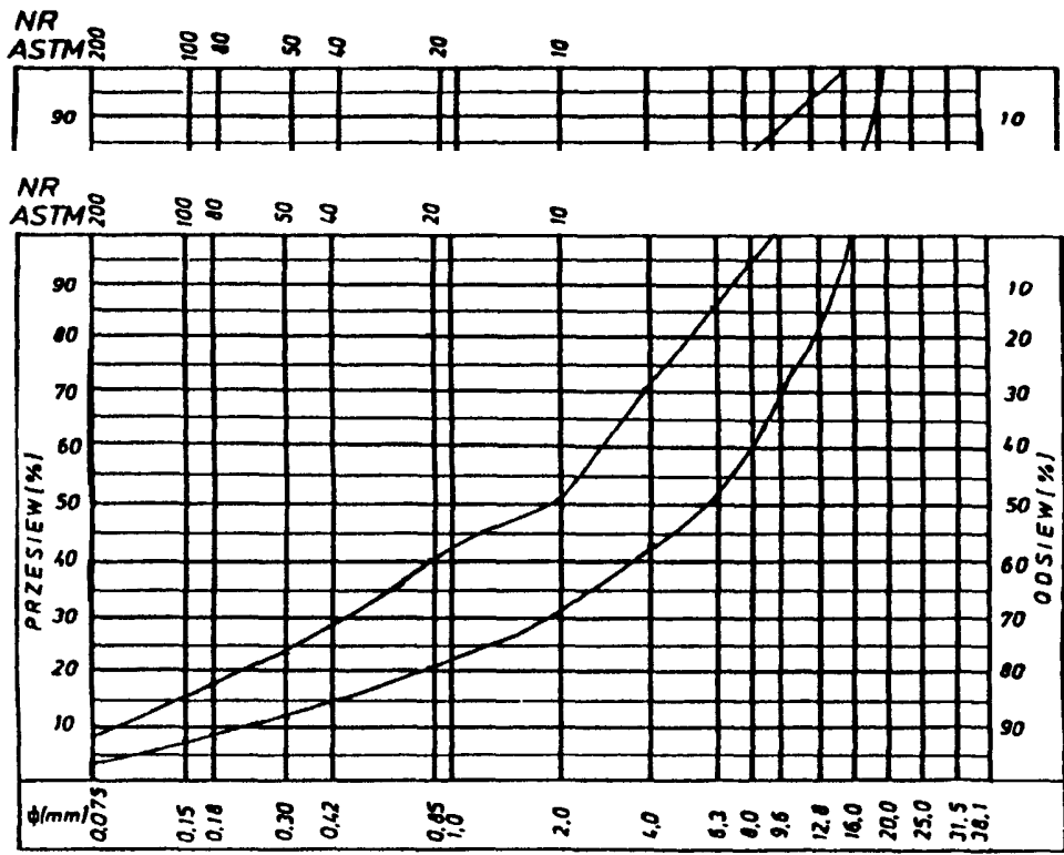
Rys. 9. Krzywe graniczne uziarnienia mieszanki mineralnej 0+16 mm do warstwy wiążącej, wyrównawczej i wzmacniającej z betonu asfaltowego dla KR 1-2
