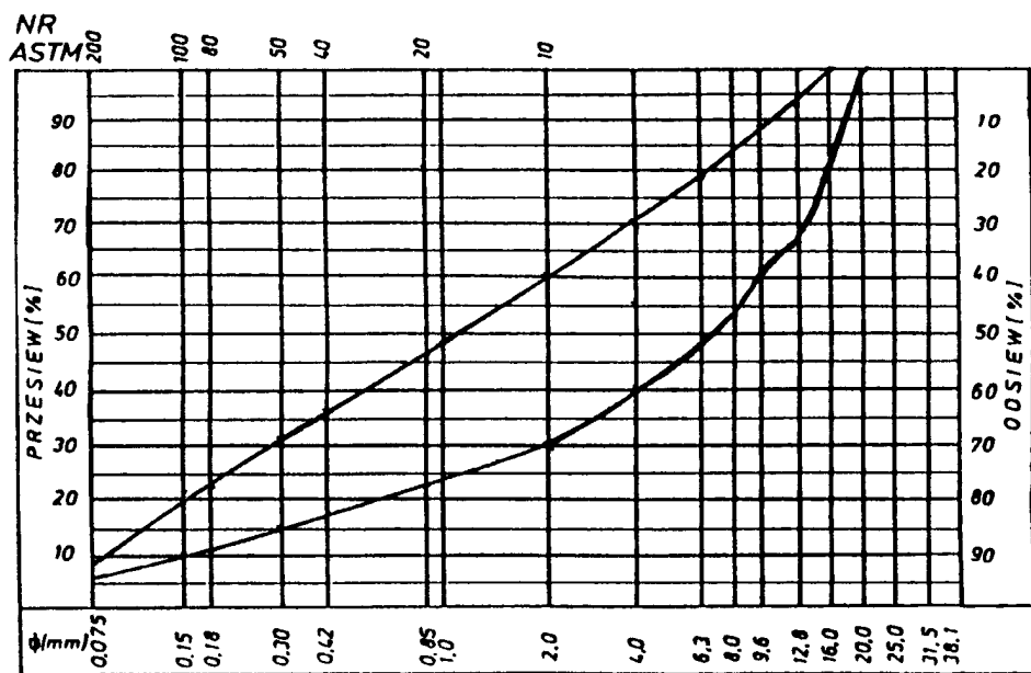
Rys. 1. Krzywe graniczne uziarnienia mieszanki mineralnej 0÷20 mm do warstwy ścierniczej z betonu asfaltowego dla KR 1-2
