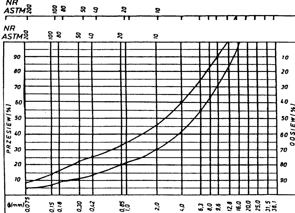
Rys. 13. Krzywe graniczne uziarnienia mieszanki mineralnej 0÷16 mm do warstwy wiążącej, wyrównawczej i wzmacniającej z betonu asfaltowego dla KR 3-6
